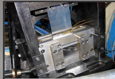
Stampo di stacco
